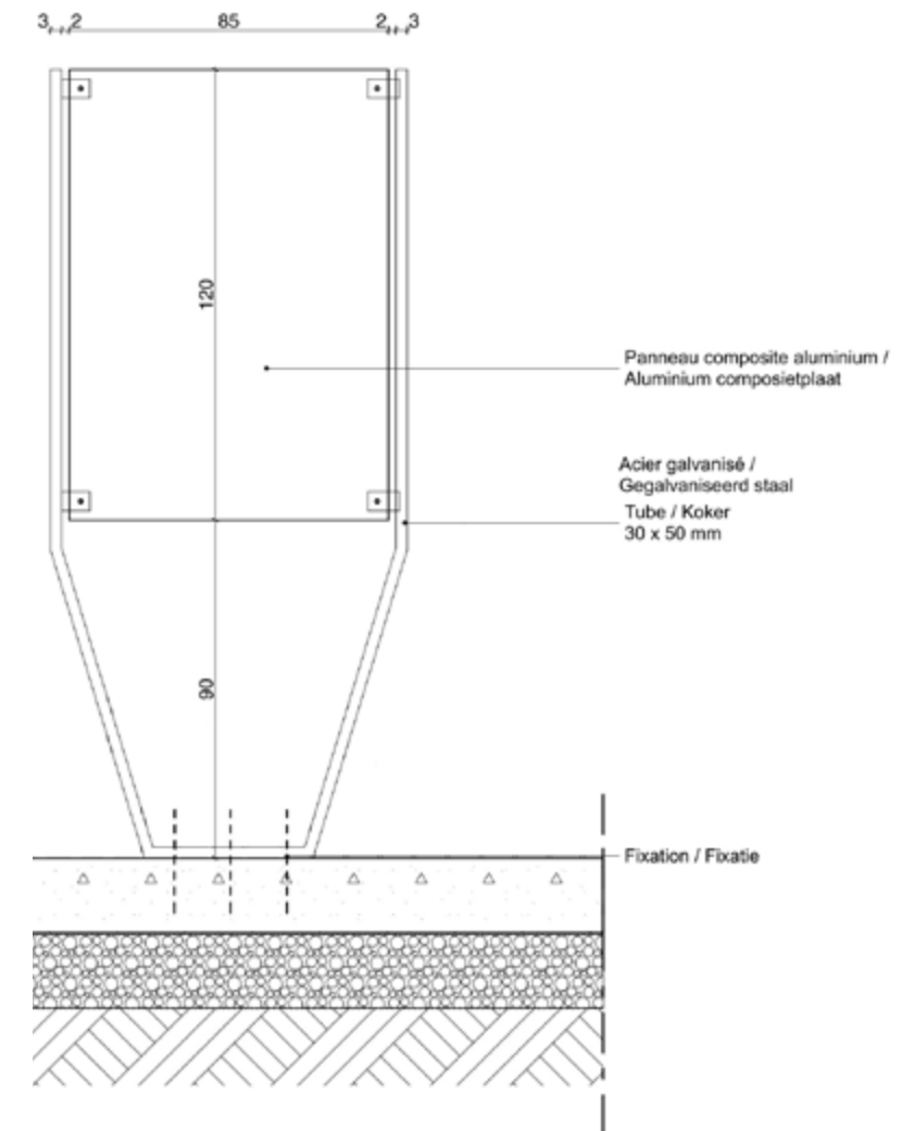
Elévation / Vooraanzicht
